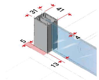
Pevný segment a boční díl
