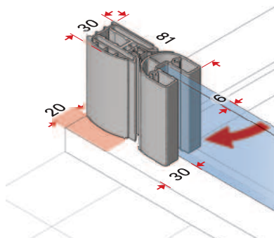
Strana pro upevnění panelu dveří
