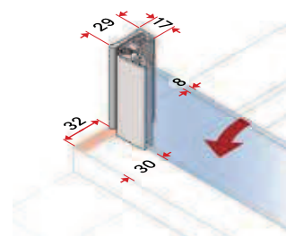
Uzavírání dveří
