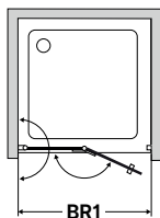
Horní pohled, upevnění vlevo
