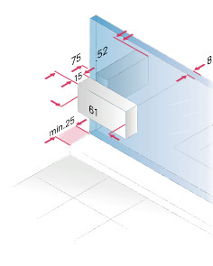
Pevný segment a boční díl
