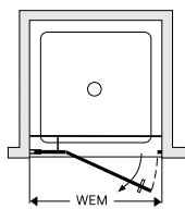
Pohled shora, upevnění vlevo
