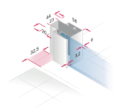
Pevný a boční segment
