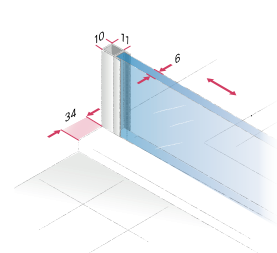
Pohled zavírání dveří
