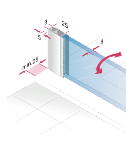
Uzavírací strana dveřního dílu
