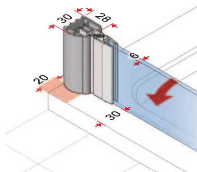
Uzavírací strana dveřního dílu
