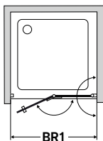
Horní pohled, upevnění vpravo
