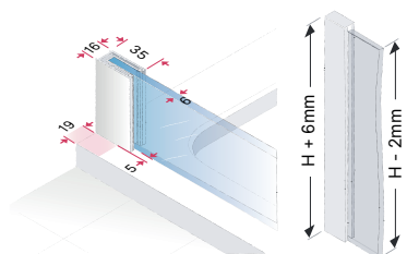
Pevný segment a boční díl
