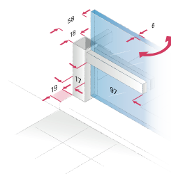
Pohled na uchytení dveří
