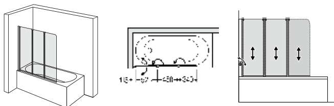
Náhled, upevnění vlevo
