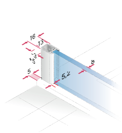
Pevný segment a boční díl
