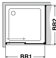
Pohled shora, panel vpravo
