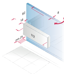
Pohled na uchycení dveří
