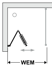
Pohled shora, upevnění vlevo, Instalace na dlažbu
