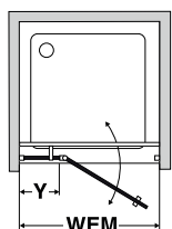
Pohled shora, uchycení vlevo
