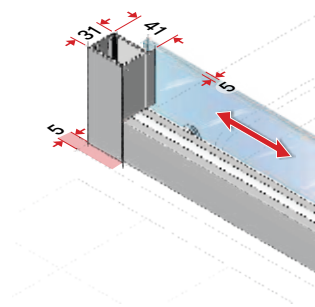
Uzavírací strana dveří
