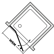
Pohled shora, upevnění vlevo
