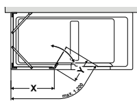
Pohled shora, upevnění vlevo
