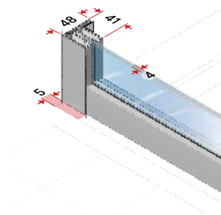
Pevný segment a boční díl
