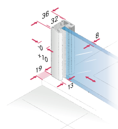
Uzavírací strana dveřního dílu
