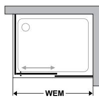
Pohled shora, dveře vlevo
