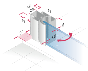
Dveřní panel, pevný segment
