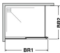
Horní pohled, upevnění vlevo
