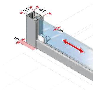
Uzavírací strana dveří, vnější pohled
