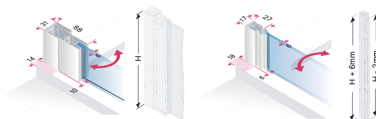
Strana pro upevnění panelu dveří
