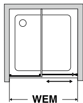
Pohled shora, upevnění vlevo
