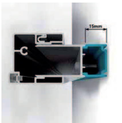
Rozšiřovací profil 508838
