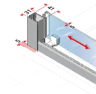
Uzavírací strana dveří, pohled zevnitř
