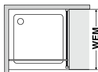
Pohled shora, upevnění vpravo
