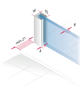
Pevný segment a boční díl s nástěnným profilem
