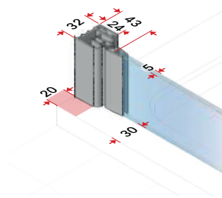
Uzavíratelná strana dveří
