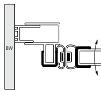
Zakončení soklovým profilem
