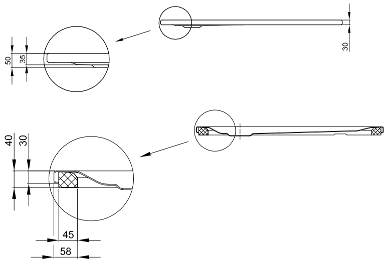
Vyobrazeno s předem namontovaným minimálním nosičem vaničky (T1).
