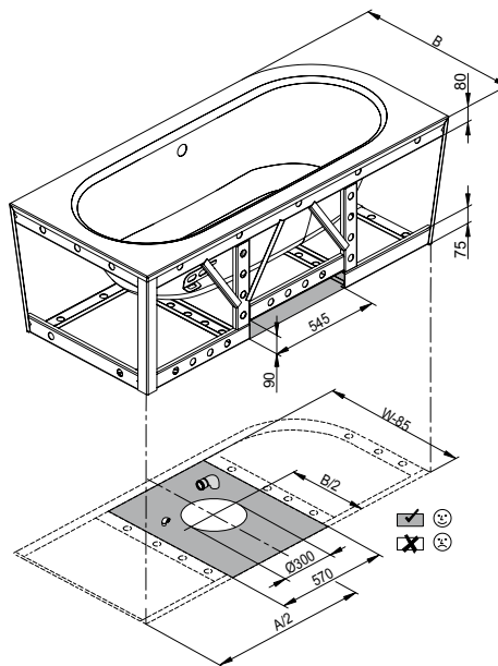
Připojovací rozměry pro odtokovou a přeřadovou soustavu
