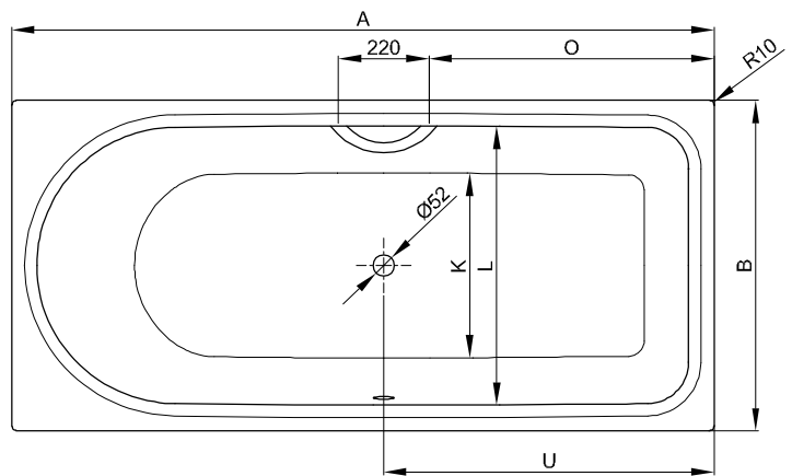
N° 2: strana nohou vpravo, přepad vpředu
