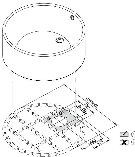
Připojovací rozměry pro odtokovou a přepadovou soustavu
