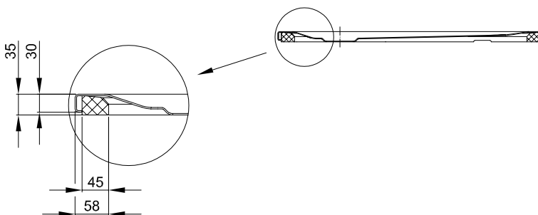
Vyobrazeno s předem namontovaným minimálním nosičem baničky (T1).
