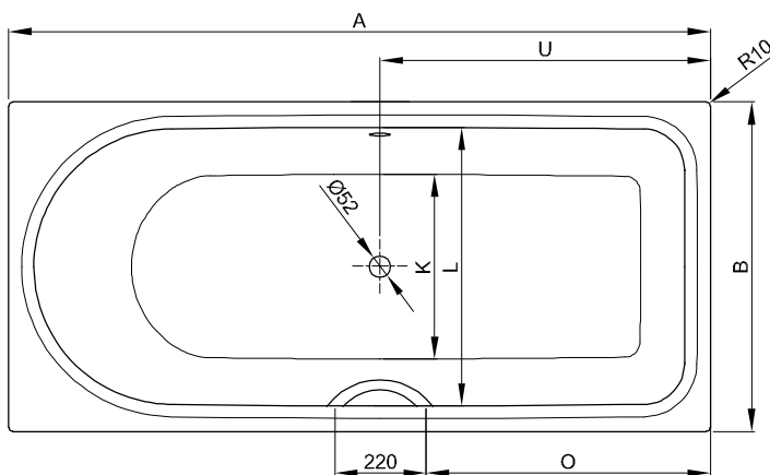
N° 1: strana nohou vpravo, přepad vzadu
