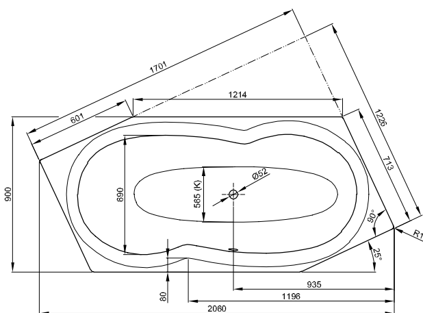
N° 1: obj. č. 6840 strana nohou vpravo, přepad vpředu
