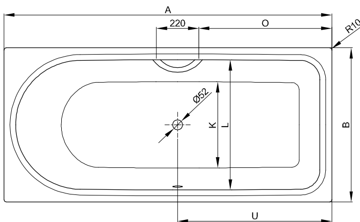
N° 2: strana nohou vpravo, přepad vpředu
