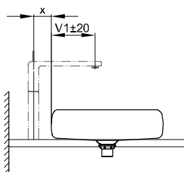
Montážní a přípojovací rozmery:
