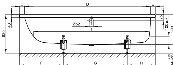
N° 2: strana nohou vpravo, přepad vpředu
