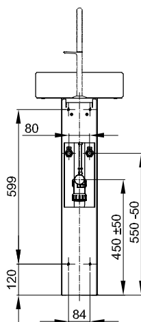
Montážní a připojovací rozměry:
