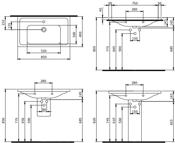
1008-001-0126 Taormina Pro Waschtisch 85cm Taormina Pro Lavabo 85 cm Taormina Pro Wastafel 85 cm
