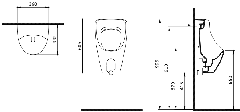
1383-001-0131 Taormina Arch Urinal Taormina Arch Urinoir Taormina Arch Urinoir
