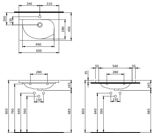
1009-001-0126 Taormina Arch Waschtisch 65 cm Taormina Arch Lavabo 65 cm Taormina Arch Wastafel 65 cm
