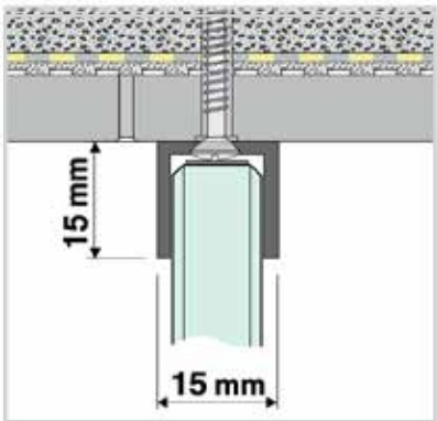
Rozměry stěnového profilu 520369 pro instalaci na obklad
