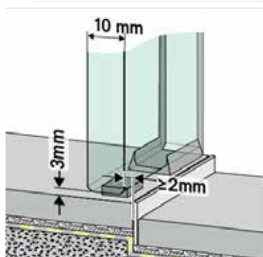
Průřez osazením skla hrany spádové lišty, upevnění vlevo
