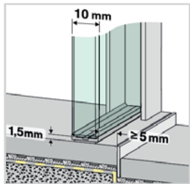
Instalace walk-in skla AIR 2 vedle hrany spádové lišty, upevnění vlevo
