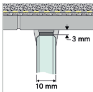
Detail bezprofilové instalace
