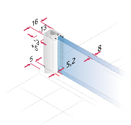
Pevný segment a boční díl
