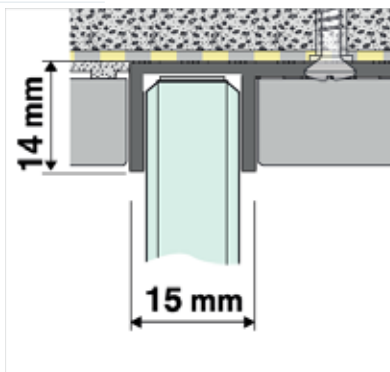
Rozměry vestavného stěnového profilu 520367 pro instalaci pod obklad
