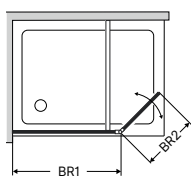
Pohled shora, upevnění vlevo
