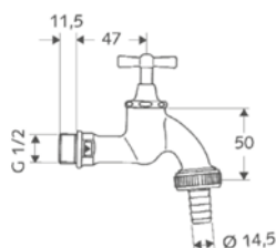
Výtokový ventil vršek s otočnou páčkou
