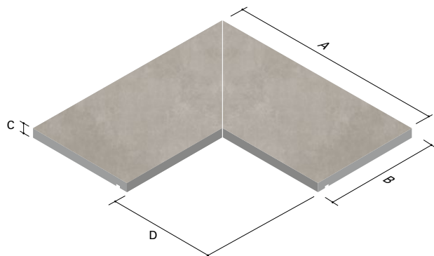
Randplatte mit Tropfkante – Innenecke (2-teilig) Border tile with drip edge - inside corner (2 pieces)
