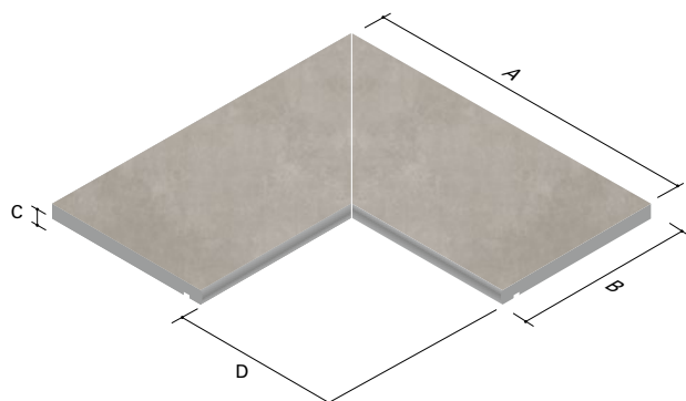
Randplatte gerundet mit Tropfkante – Innenecke (2-teilig) Border tile, rounded, with drip edge - inside corner (2 pieces)
