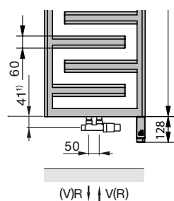
Elektrická prevádzka: s vstavanou el. vyk. tyčou IHC
