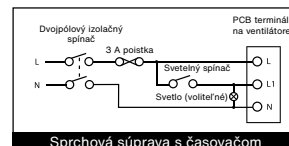
Schéma zapojenia
