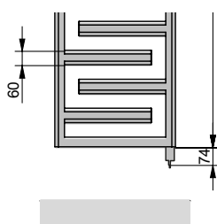
Elektrická prevádzka: s vstavanou el. vyk. tyčou IHD
