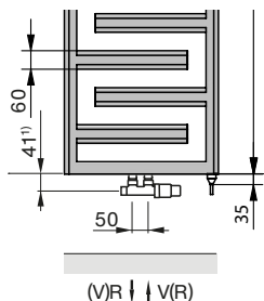
Elektrická prevádzka: s vstavanou el. vyk. tyčou IHE
